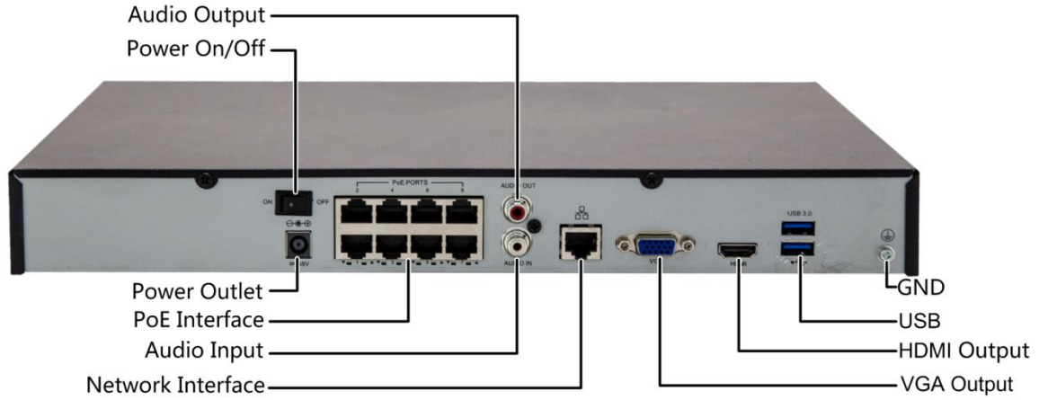
NVR201-08EP
